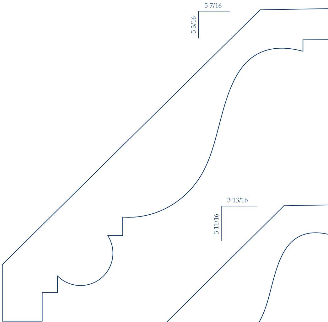
IL 385 1 5/16 x 7 1/2
