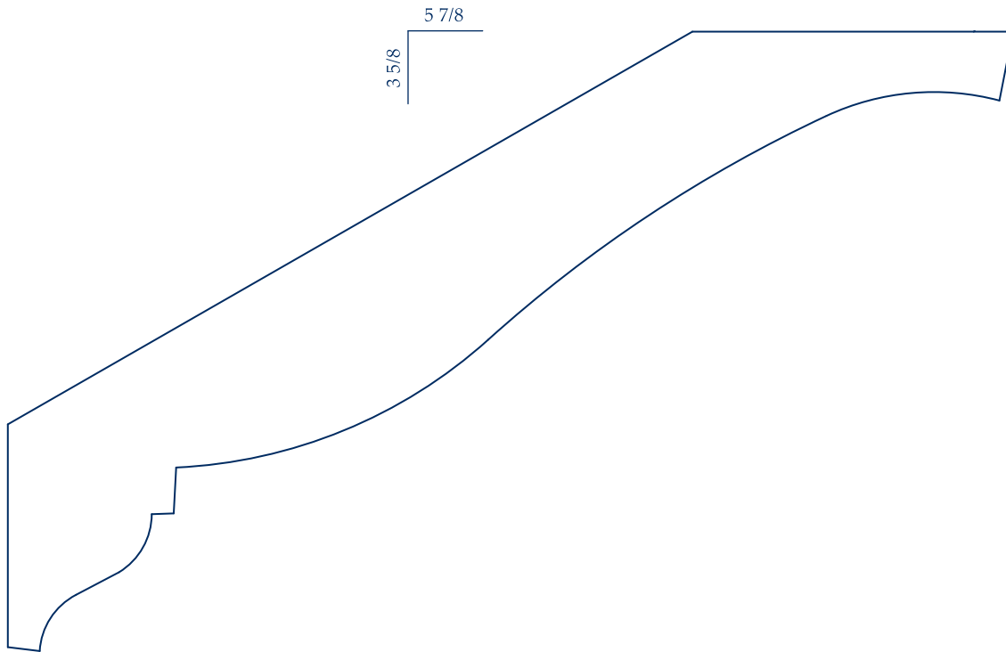
IL 327 1 1/4 x 6 7/8
