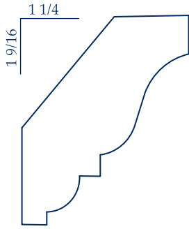
IL 310 1 1/16 x 2
