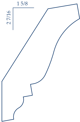
IL 313 1 1/16 x 2 7/8
