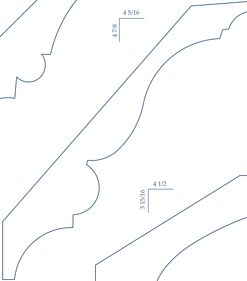
IL 356 1 x 6 1/2
