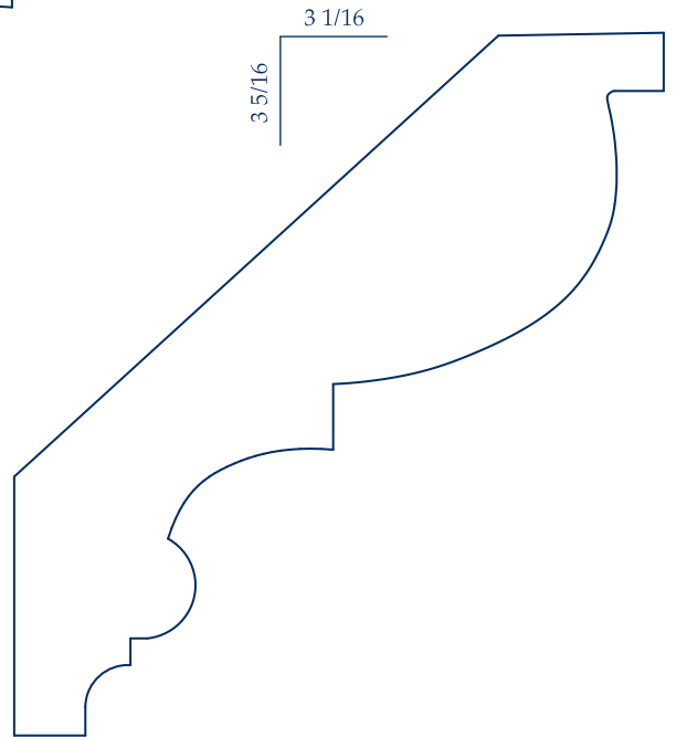
IL 380 1 1/8 x 4 1/2
